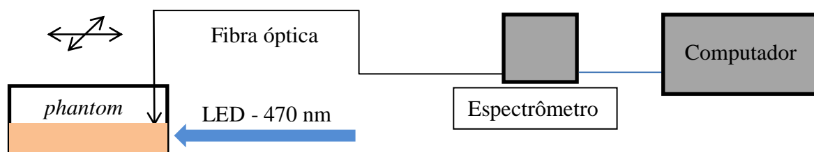
Figura 21: Arranjo experimental para medidas de Penetração e Espalhamento de luz em Phantoms das soluções aquosas de leite.
