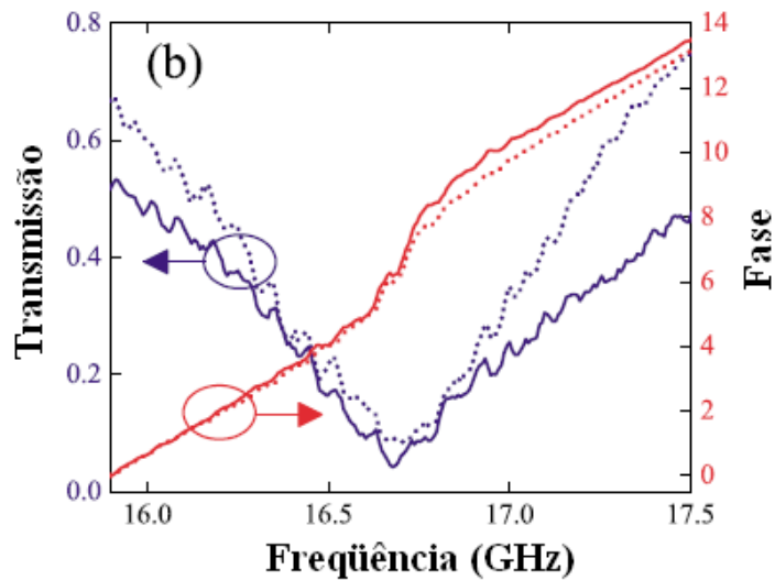
Figura 1.15: Gráfico da transmissão e da fase para \beta = 50^\circ . As linhas cheias correspondem aos resultados experimentais e as linhas pontilhadas aos calculados [12].
