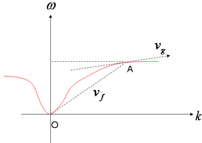
Figura 1.3: Curva de dispersão.
