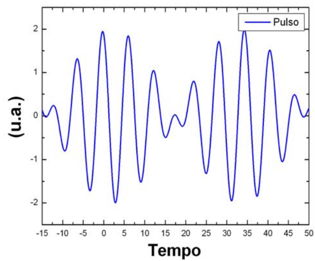
Figura 1.2: Onda resultante da combinação de duas ondas com diferentes frequências e mesma amplitude.
