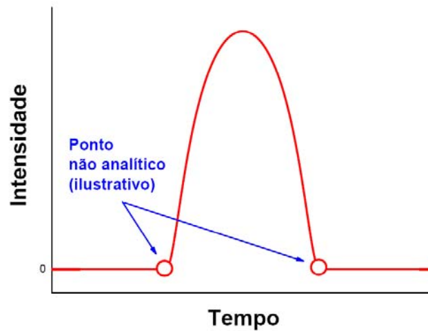
Figura 3.8: Esquema de um pulso com suporte compacto.
