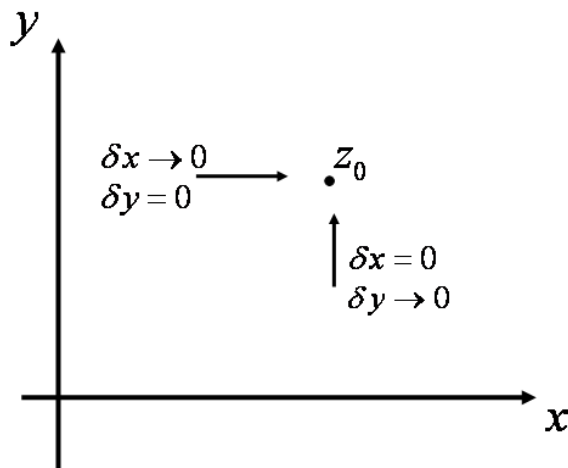
Figura 2.2: Esquema mostrando as duas formas de aproximação escolhidas para demonstração das relações de Cauchy-Riemann.
