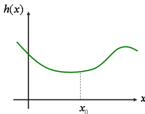
Figura 2.4: Esquema de uma função analítica.
