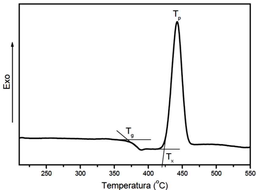
Figura 2.3: Análise térmica exploratória do \text{PbGeO}_3 .
