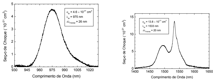
Figura 4.12: Espectros das seções de choque de absorção em função do comprimento de onda, para a amostra PZABP dopada com \text{Er}^{3+} e \text{Er}^{3+}/\text{Yb}^{3+} para as bandas de 980 nm e 1530 nm.
