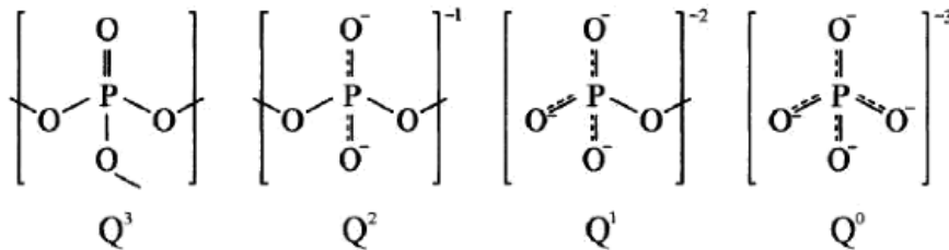
Figura 2.4: Unidades estruturais básicas formadas por tetraedros [PO_4] nos vidros de fosfato.
