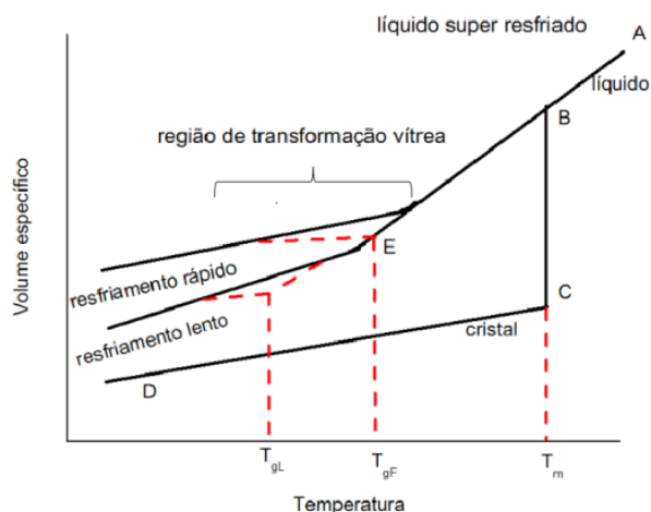
Figura 2.2: Definição da temperatura vítrea.
