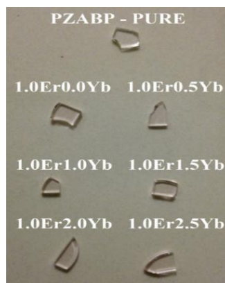
Foto 4.1: Amostras PZABP preparadas com corte e polimento para as medidas.
