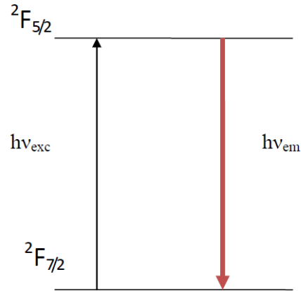
Figura 2.10: Diagrama parcial de níveis de energia do íon Yb^{3+} .
