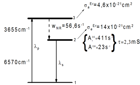
Figura 4.15: Níveis de energia com alguns parâmetros, indicando as rotas de relaxação para os estados {}^4I_{11/2} - {}^4I_{13/2} (980nm) e {}^4I_{13/2} - {}^4I_{15/2} (1530nm) que são os que apresentam maior relevância.
