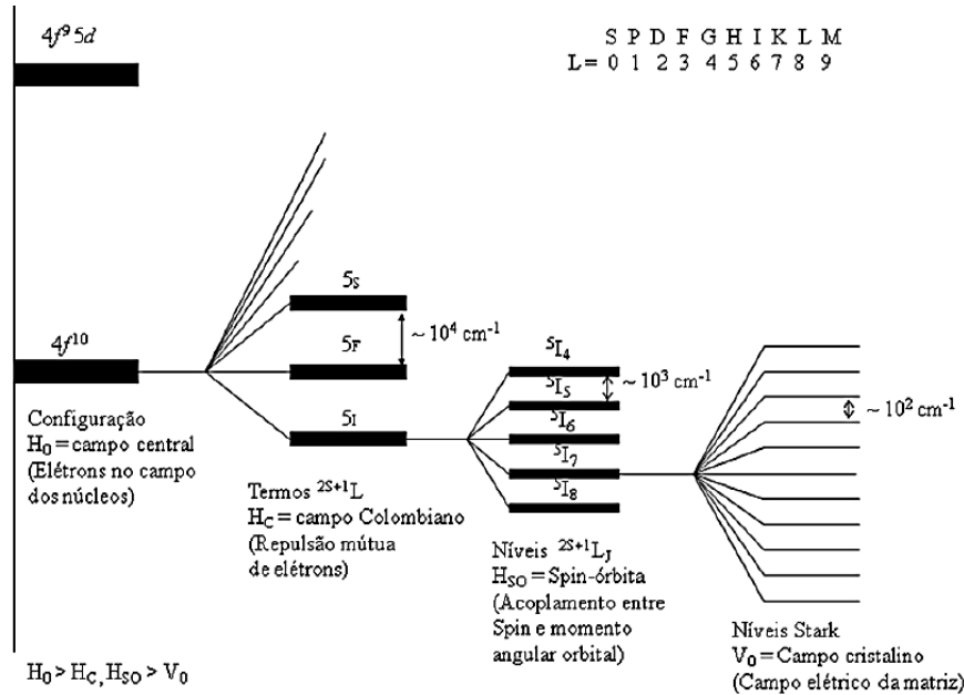
Figura 2.7: Desdobramentos dos níveis de energia dos íons terras raras quando esses são submetidos a um campo cristalino.
