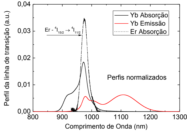
Figura 4.14: Perfil de linha de transição em função do comprimento de onda, mostrando a seção de choque de emissão do \text{Yb}_2\text{O}_3 .
