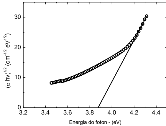
Figura 4.10: Relação de (\alpha E)^{1/2} em função de h\nu para a matriz vítrea PZABP pura, com ajuste linear da energia de separação óptica.
