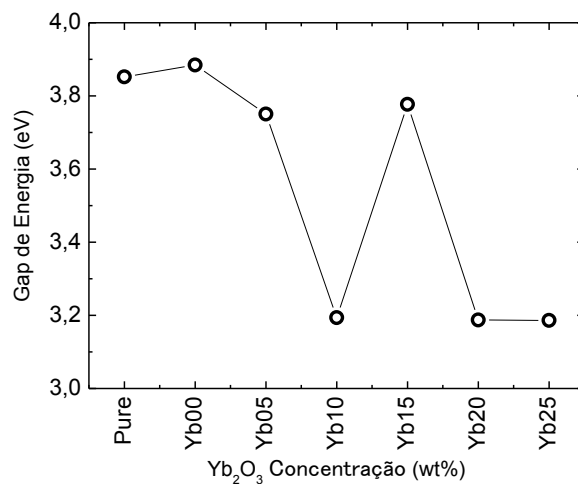
Figura 4.11: Energia de gap transformada de comprimento de onda em eV em função da concentração de \text{Yb}_2\text{O}_3 . A dopagem de \text{Er}_2\text{O}_3 foi mantida constante em 1,0 wt% em todas as amostras, exceto na pura.
