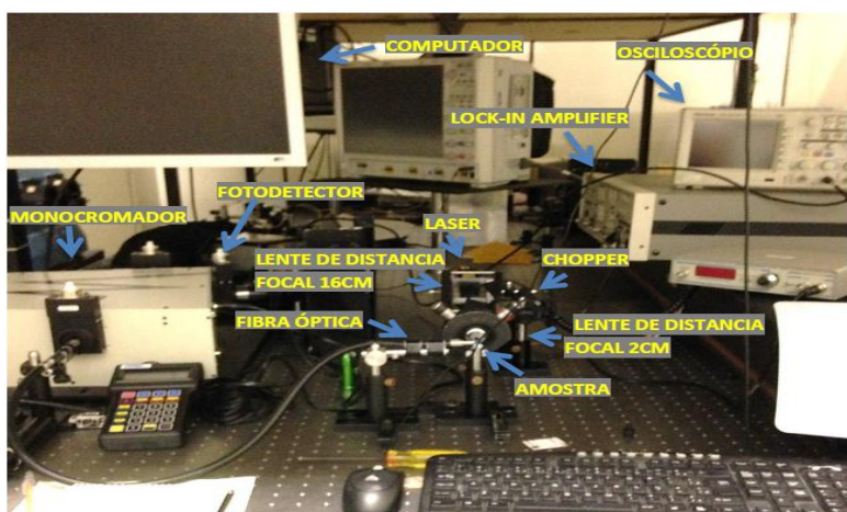
Figura 3.6: Aparato experimental do tempo de vida.
