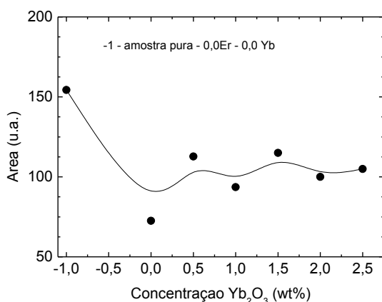
Figura 4.8: Área da região IV (2000 nm a 3000 nm) do vidro PZABP para os comprimentos de onda das amostras pura, dopada com \text{Er}_2\text{O}_3 em 1,0 % em peso e codopadas com \text{Yb}_2\text{O}_3 de 0 a 2,5
