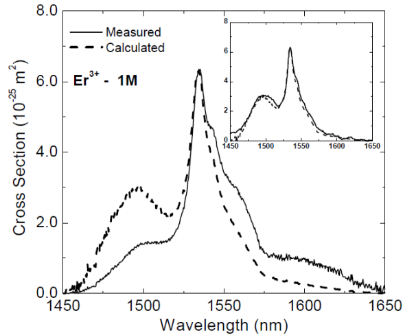
Figura 2.14: Seção transversal determinada pela teoria McCumber (Absorção calculada - curva a tracejado, e a medição experimental da banda de absorção).
