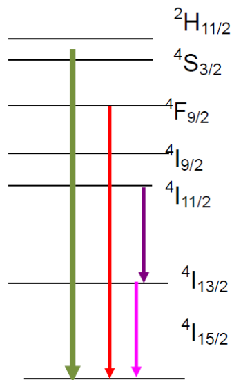
Figura 2.8: Diagrama parcial de níveis de energia do íon érbio indicando transições características.
