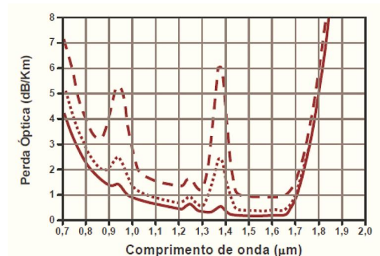
Figura 2.9: Perda óptica em função do comprimento de onda para vidros silicatos.
