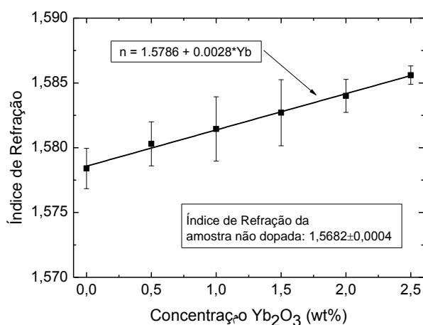
Figura 4.3: Índice de refração do vidro PZABP em função da concentração de \text{Yb}_2\text{O}_3 . A dopagem de \text{Er}_2\text{O}_3 foi mantida constante em 1,0 wt% em todas as amostras, exceto na pura.
