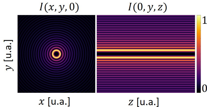
Figura 2.6: Distribuição de intensidade e perfil da propagação de um feixe Bessel de ordem m = 4 .
