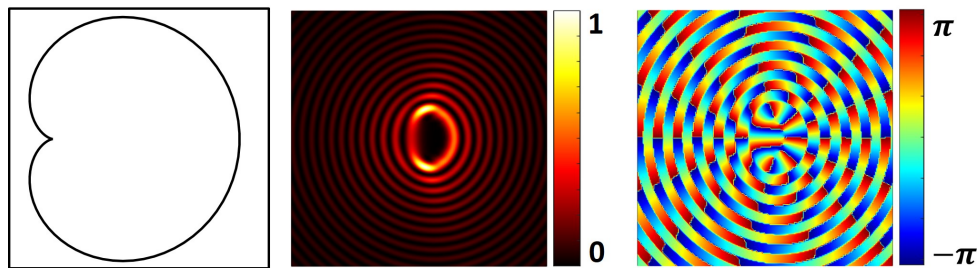
Figura 3.5: Feixe gerado a partir da parametrização de um cardioide com m = 7 e para um vetor de onda transversal k_t = 12\pi \text{ mm}^{-1} .
