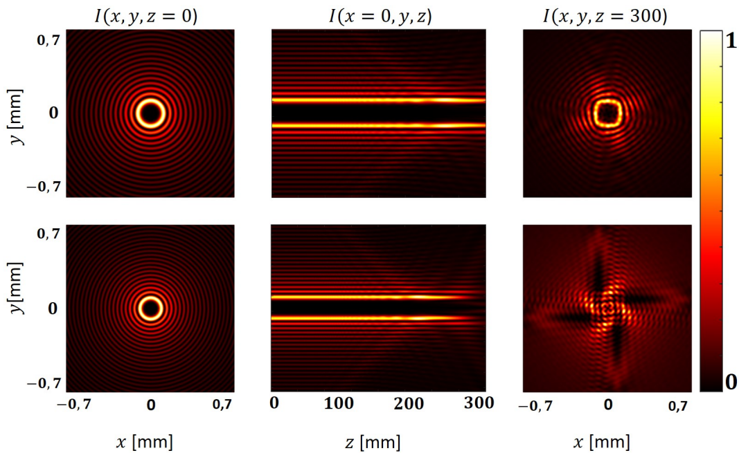
Figura 3.8: Padrões de intensidade e perfil da propagação para feixes circulares com componentes transversas do vetor de onda k_t = 10\pi \text{ mm}^{-1} e k_t = 12\pi \text{ mm}^{-1} , respectivamente.
