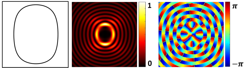
Figura 3.4: Feixe gerado a partir da parametrização de uma curva seno oval com m = 7 e para um vetor de onda transversal k_t = 12\pi \text{ mm}^{-1} .
