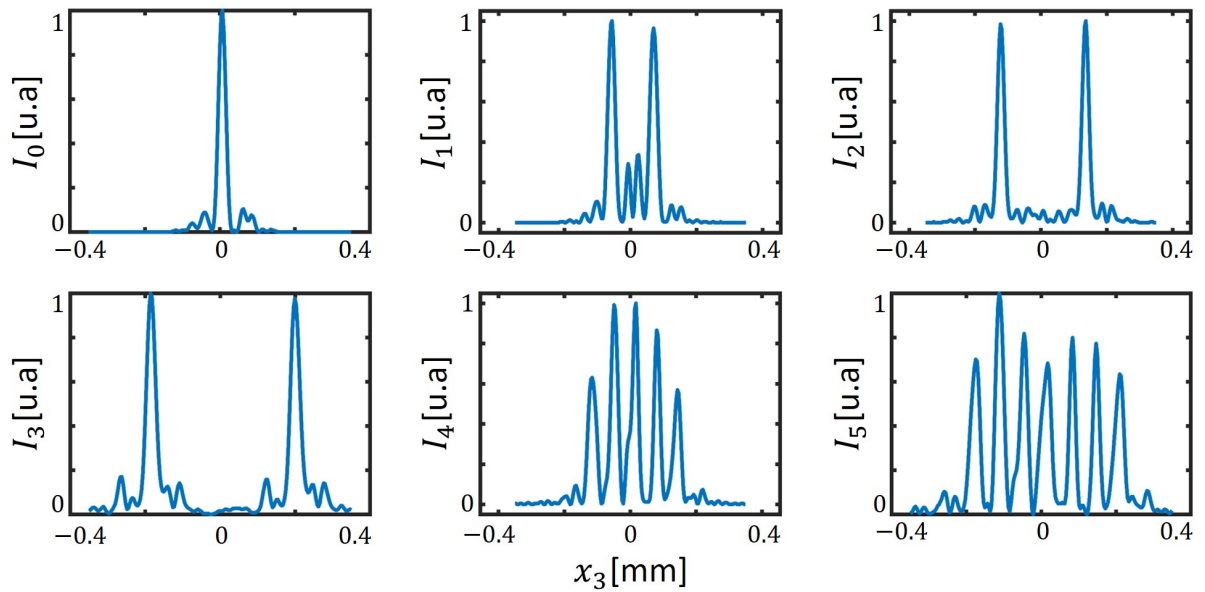
Figura 5.15: Exibição dos respectivos perfis horizontais ao longo das linhas médias tracejadas da Fig.5.14.
