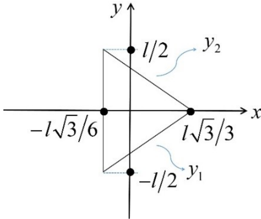
Figura 4.5: Geometria da borda de uma abertura triangular equilátera com lados de comprimento l . y_1 e y_2 representam funções lineares que descrevem as bordas da abertura triangular, como indicado pelas setas.
