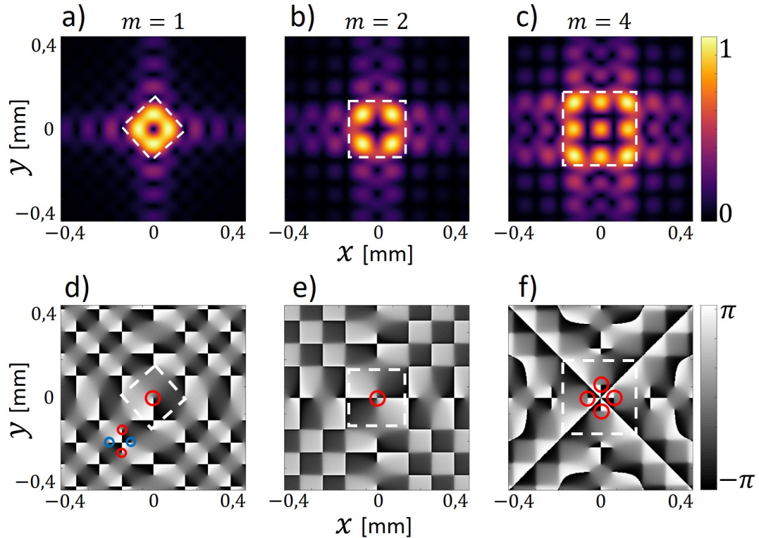
Figura 4.9: Da mesma maneira que na Fig.(4.7), aqui temos feixes Laguerre-Gauss de alta ordem difratado por aberturas quadradas, na zona de Fraunhofer, obtido por cálculo analítico. Em (a), (b) e (c) é exibido as distribuição transversa de amplitude. As imagens (d), (e) e (f) mostram as distribuições de fase.
