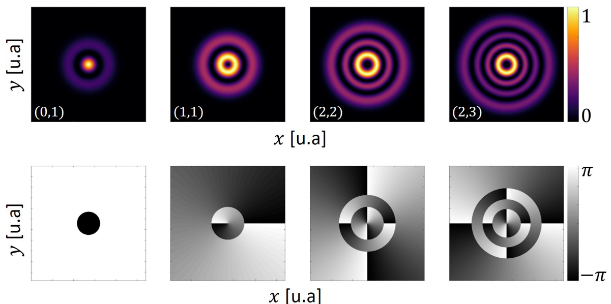
Figura 2.1: Representação dos padrões de intensidade para modos Laguerre-Gauss de diferentes índices azimutal e radial. Cada modo é identificado pelo par (m, p) .
