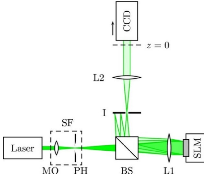
Figura 3.7: Configuração experimental composta das lentes L1 e L2 ; de um filtro espacial (FE) composto de uma lente objetiva microscópica (OM) e um furinho (P) de 50 \mu\text{m} de diâmetro; de um divisor de feixe (BS); uma íris (I); um modulador espacial de luz (Spatial Light Modulator, SLM); e de uma câmera CCD acoplada a um dispositivo que a translada.
