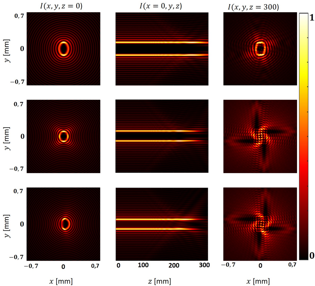
Figura 3.9: Padrão de intensidade e perfil da propagação para um feixes elíptico, cardioide e seno oval.
