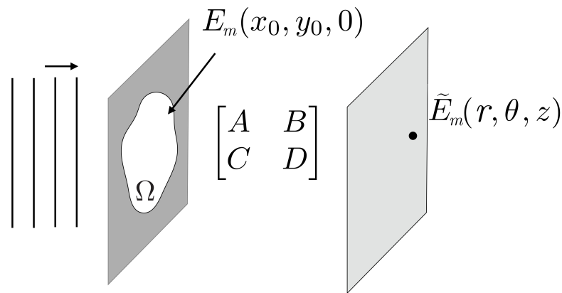
Figura 4.4: Geometria do sistema. O feixe de luz E_m , depois de cruzar a abertura \Omega , difrata através de um sistema ABCD produzindo o campo final \tilde{E}_m .
