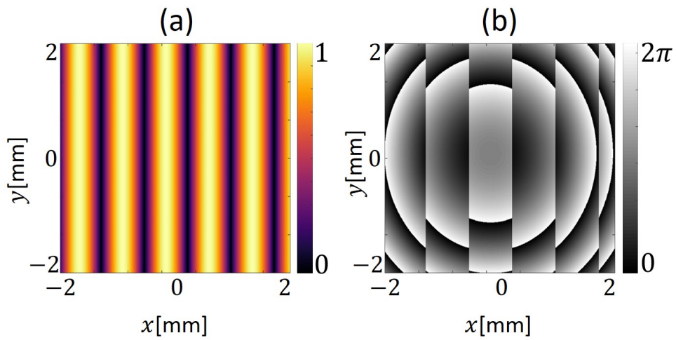
Figura 2.16: Em (a), é exibido o padrão de intensidade e em (b) a distribuição de fase do experimento de Young de dois furos.
