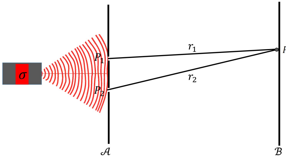
Figura 6.1: Notação relacionada ao experimento de interferência de Young, a partir do qual as funções de correlação de segunda ordem de um feixe de luz podem ser determinadas.
