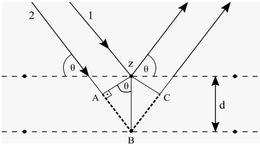
Figura 4.1 – Derivação da lei de Bragg para difração de raios x.
