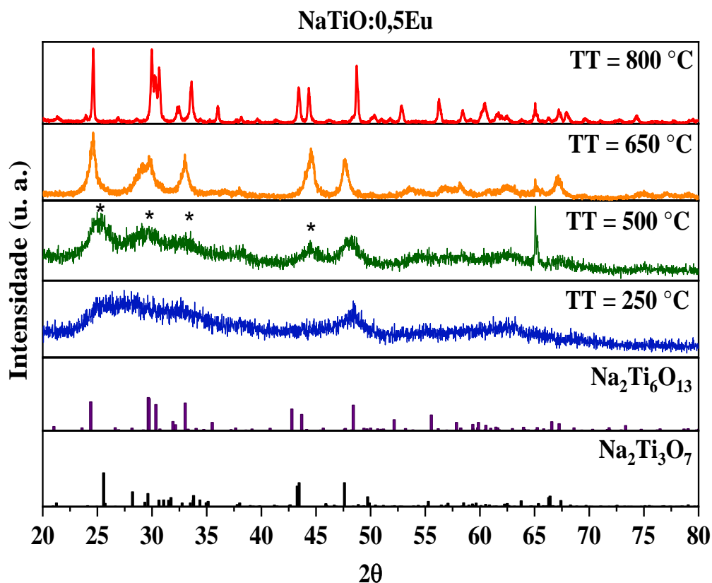
Figura 5.2 – Difratoogramas de raios-X das amostras de NaTiO:0,5Eu submetidas a quatro temperaturas de tratamentos térmicos (TT): 250 °C, 500 °C, 650 °C e 800 °C. Também está incluído o padrão cristalográfico referente as fases Na 2 Ti 3 O 7 (Trititanato de Sódio, JCPDS Card 47-0124) e Na 2 Ti 6 O 13 (Hexatitanato de sódio, JCPDS Card 73-1398).
