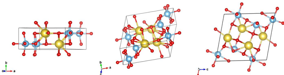
Figura 2.4 – Estrutura cristalina do \text{Na}_2\text{Ti}_3\text{O}_7 vista por alguns ângulos.
