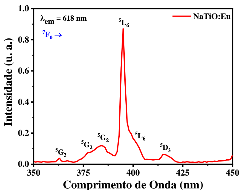
Figura 6.1 – Espectro de excitação da amostra de \text{NaTiO:5Eu} na região de 350 a 450 nm, referente à emissão em 618 nm. Amostra tratada termicamente a 500°C.
