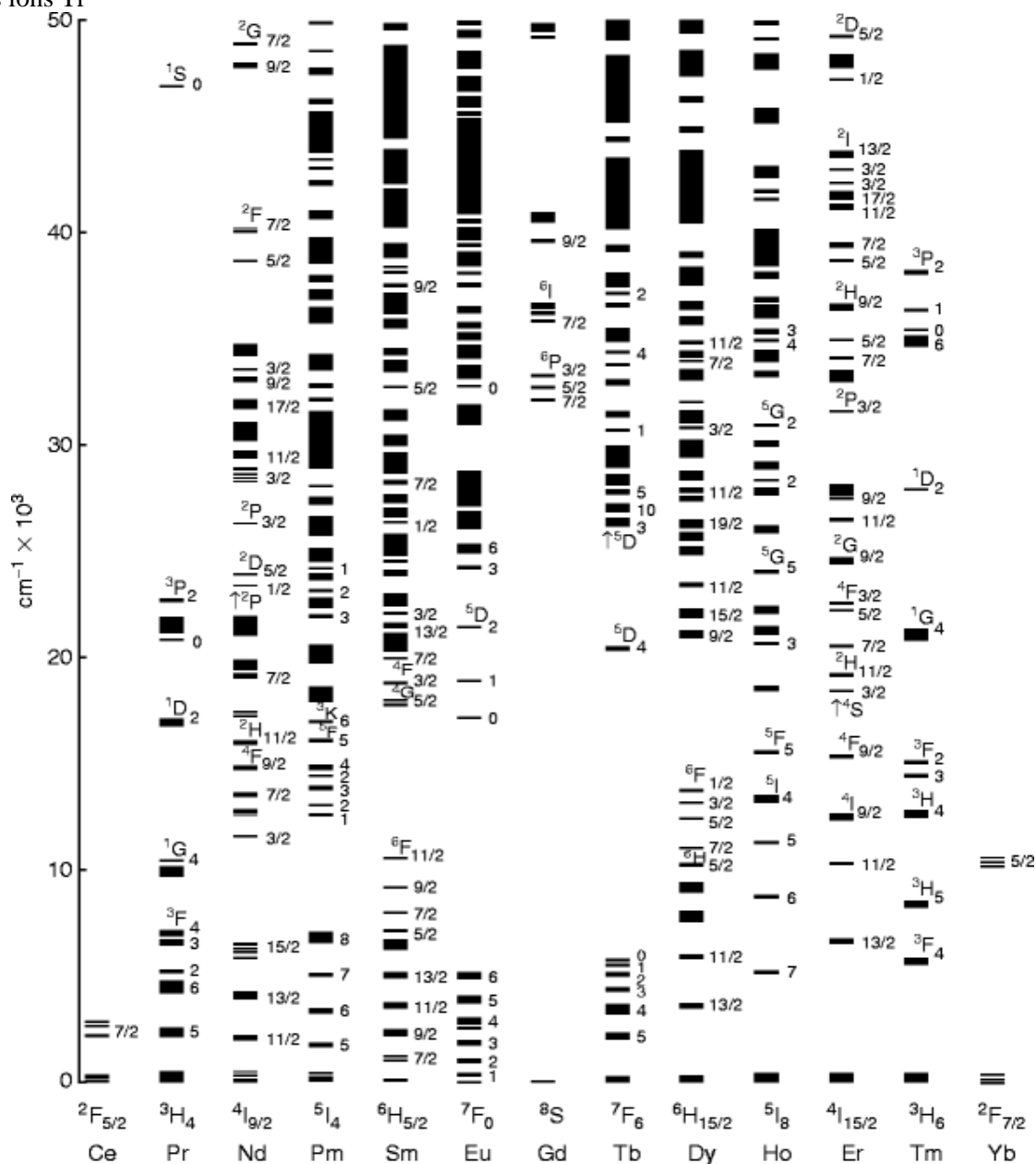
Figura 1.2 – Diagrama de níveis elaborado por Dieke e colaboradores referentes aos níveis energéticos dos íons \text{Tr}^{3+} .
