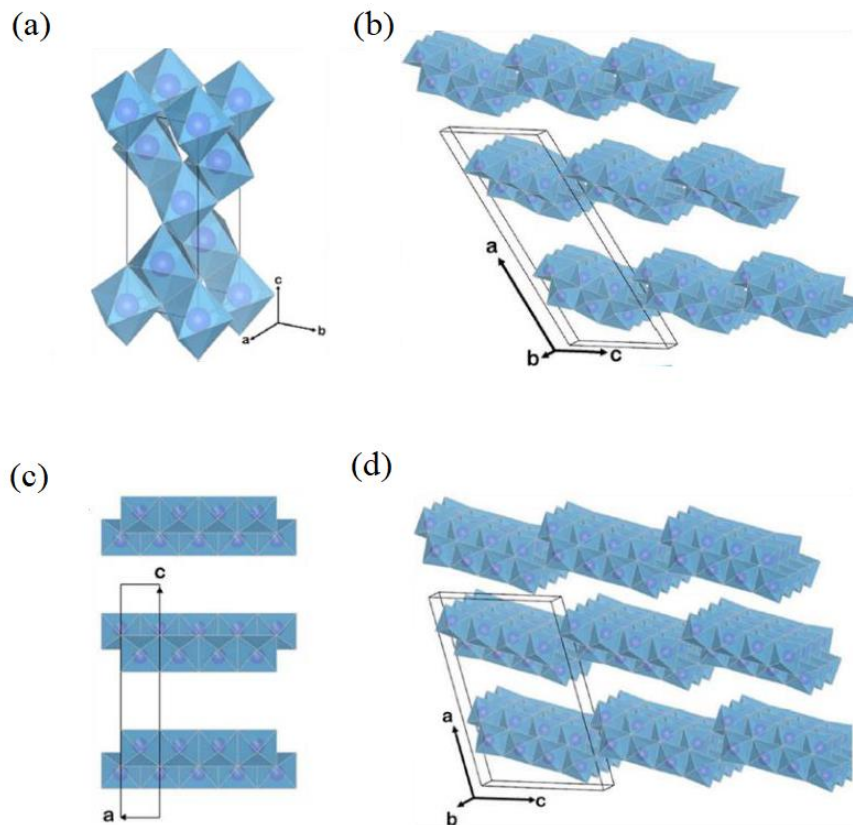
Figura 2.2 – Estrutura cristalina destacando as unidades octaédricas de \text{TiO}_6 do a) \text{TiO}_2 anatase, b) \text{H}_2\text{Ti}_3\text{O}_7 monoclínico, c) \text{H}_2\text{Ti}_4\text{O}_9 monoclínico e d) \text{H}_2\text{Ti}_4\text{O}_9 ortorrômbico.
