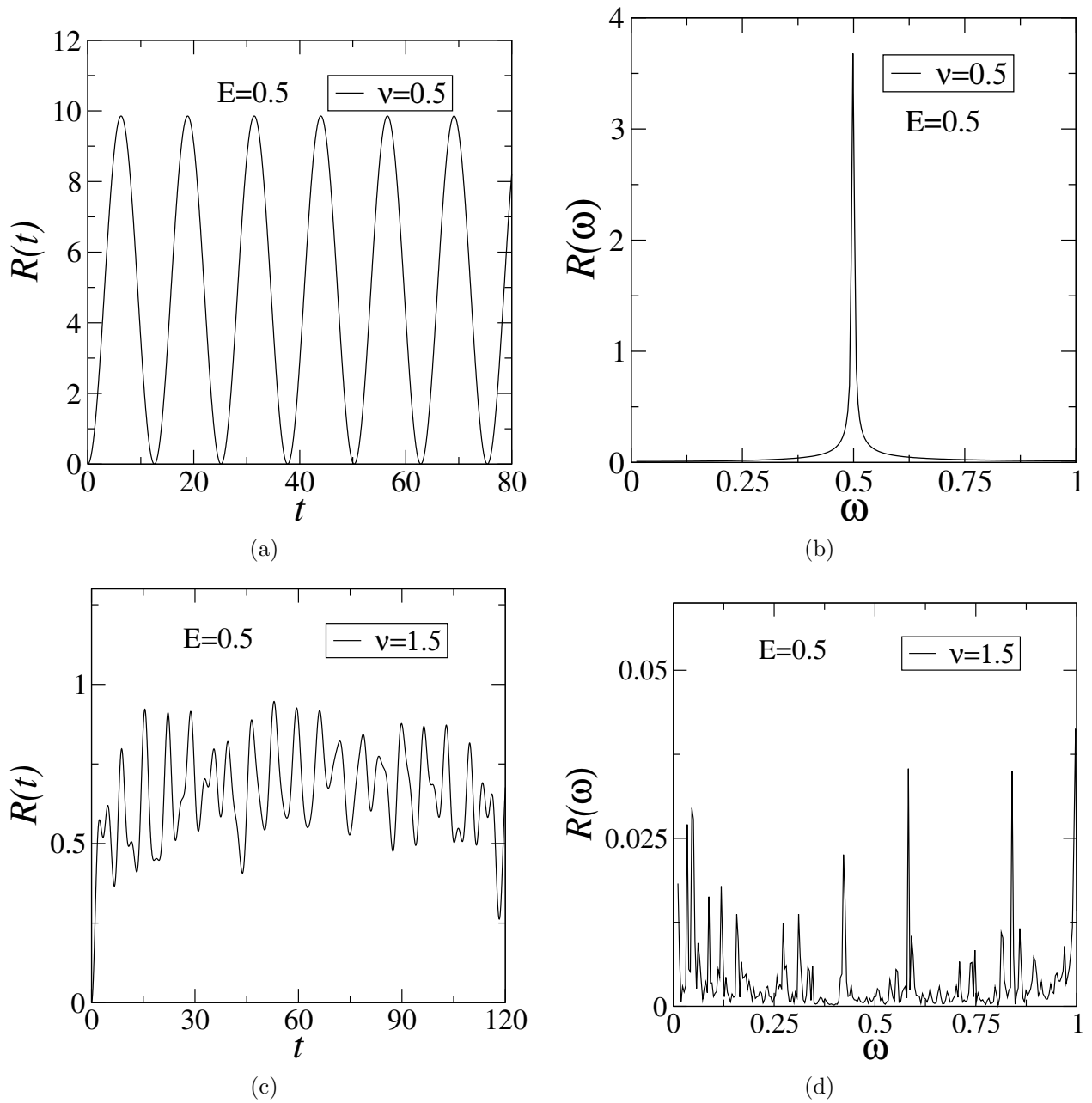
Figura 3.2: (a), (c) Posição média eletrônica R(t) versus t para E_x = E_y = E = 0.5 com \nu = 0.5 e 1.5. (b),(d) A transformada de Fourier R(\omega) versus \omega para os respectivos casos (a) e (b).
