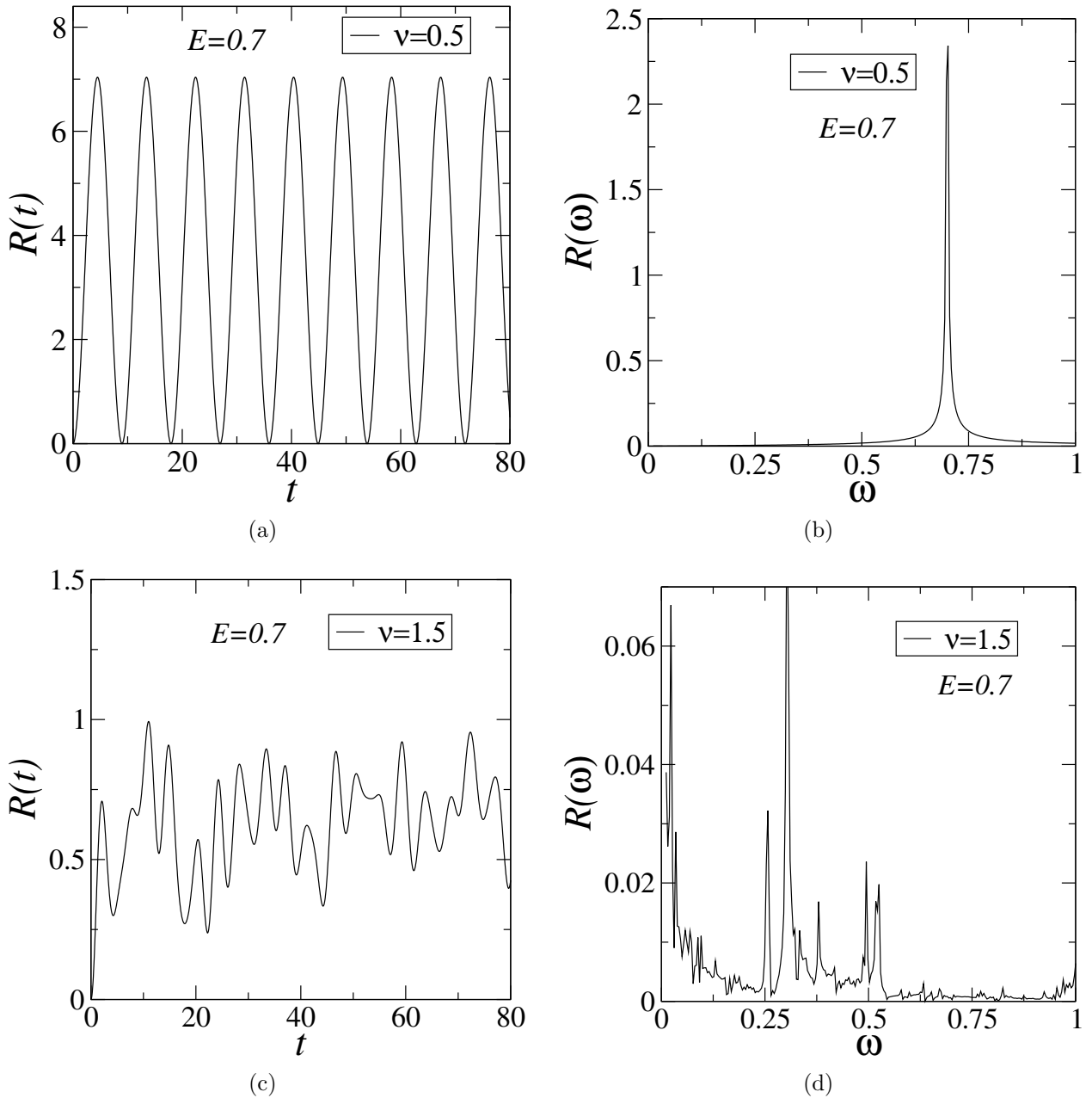
Figura 3.3: (a), (c) Posição média eletrônica R(t) versus t para E_x = E_y = E = 0.7 com \nu = 0.5 e 1.5. (b),(d) A transformada de Fourier R(\omega) versus \omega para os respectivos casos (a) e (b).
