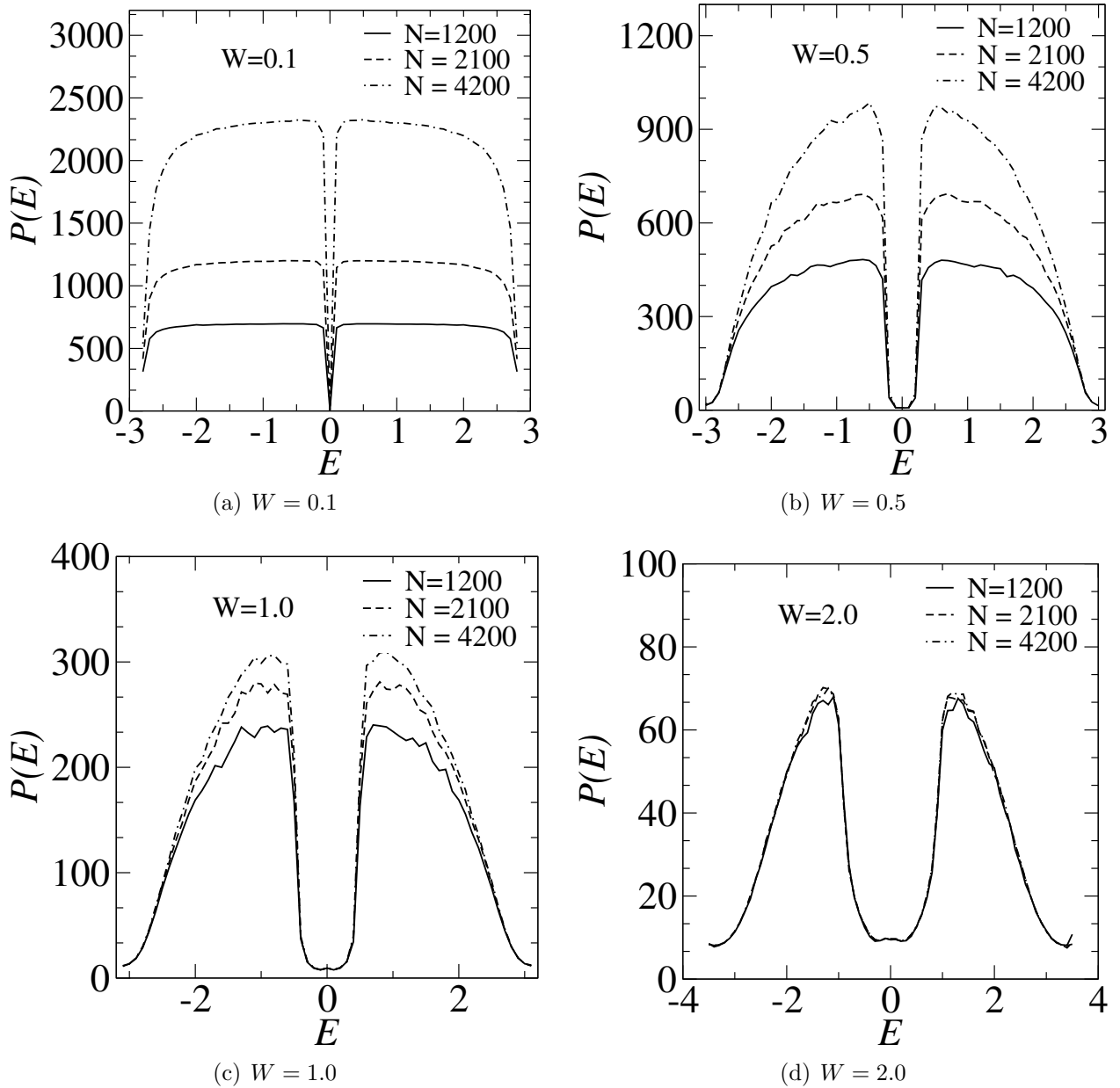
Figura 5.3: (a-d) O número de participação P(E) versus energia E para W = 0.1, 0.5, 1.0, 2.0 e N = 1200, 2100, 4200 .
