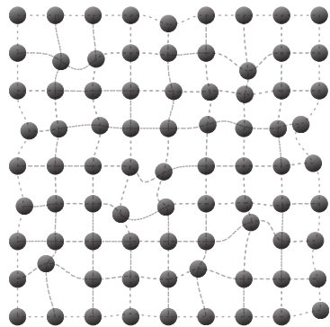
(d) Rede com deslocamento (desordem estrutural).
