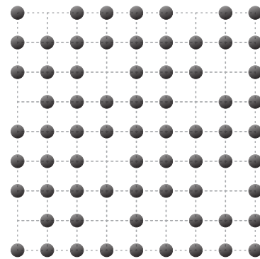
(b) Rede com desordem composicional do tipo lacunas ou vacância.
