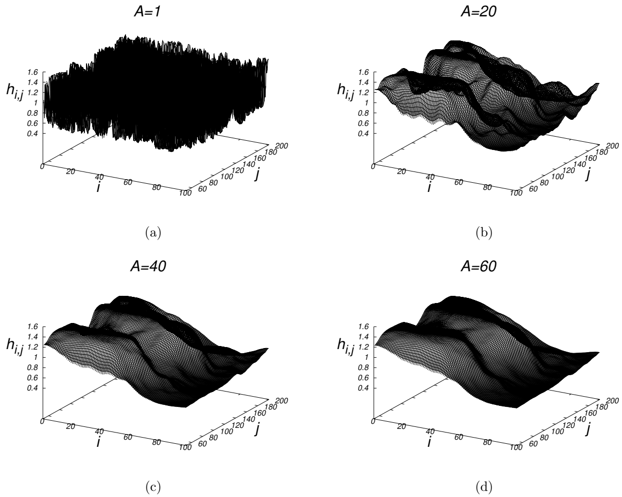
Figura 4.1: Perfil de hopping completo h_{i,j} versus i e j para A = 1, 20, 40, 60 .
