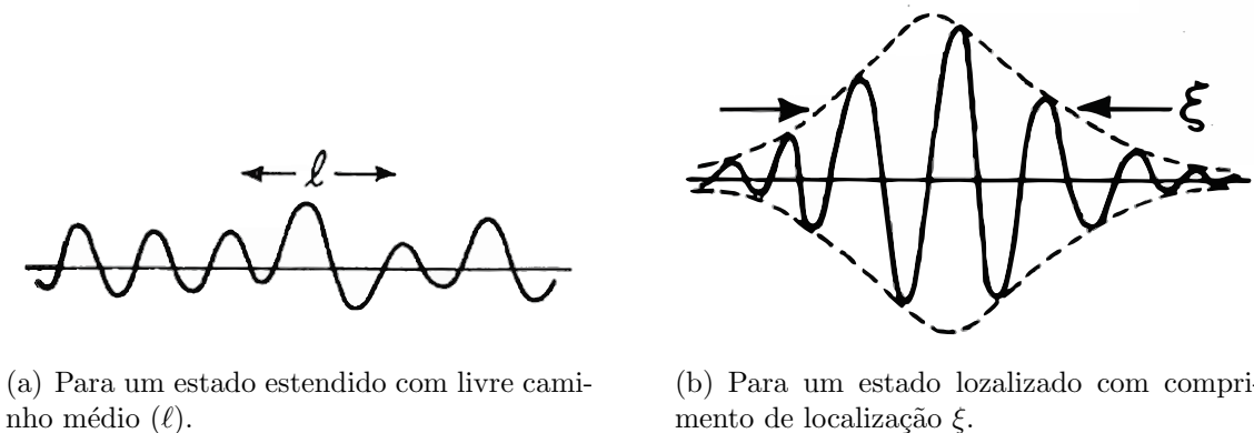
Figura 2.3: Representação da função de onda típica.
