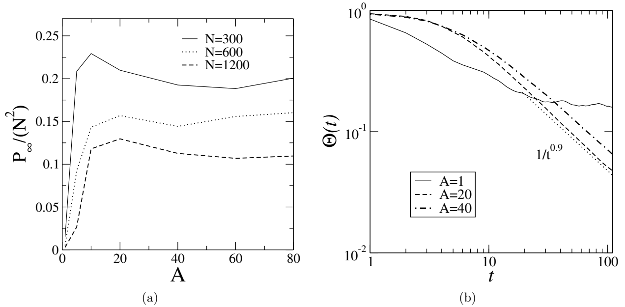
Figura 4.3: (a) O número de participação redimensionado para tempo longo P_\infty/N^2 = P(t \rightarrow \infty)/N^2 versus A para N = 300 até 1200. (b) A função de autocorrelação temporal \Theta(t) para A = 1, 20, 40 .
