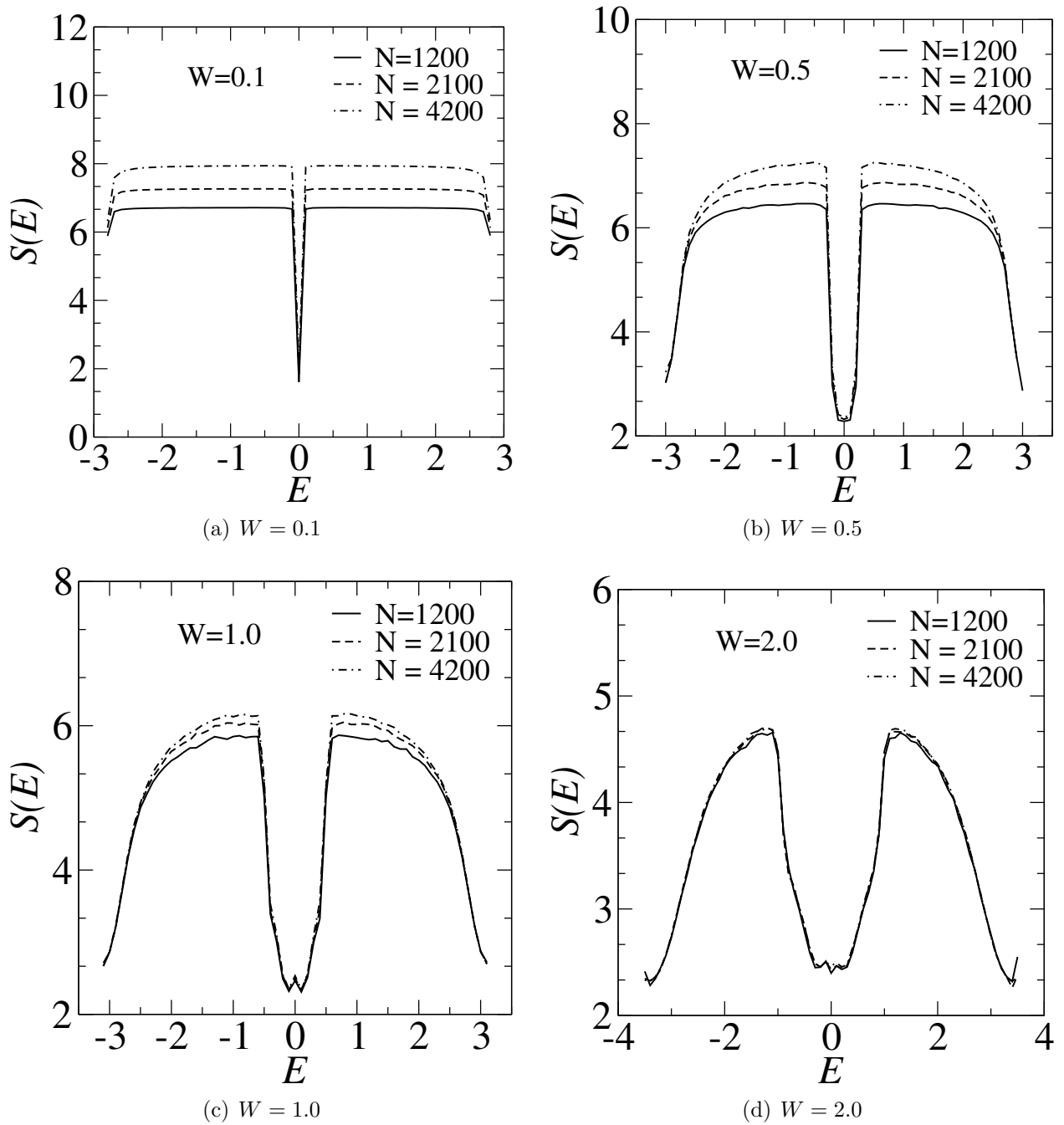
Figura 5.4: (a-d) A entropia de Shannon S(E) versus energia E para W = 0.1, 0.5, 1.0, 2.0 e N = 1200, 2100, 4200 . Esse resultados estão em boa concordância com os mostrados na Figura 5.3, onde todos os autoestados permanecem localizados.
