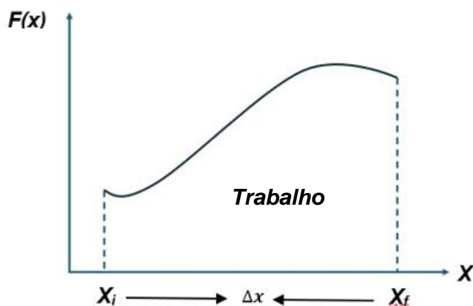
Figura 4.2: Força variável em função da posição de um corpo se movendo na direção x . O trabalho realizado pela força é numericamente igual à área sob o gráfico da força em relação à posição.
