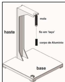
Figura 13 - Imagem da prova experimental da OBFEP 2014
