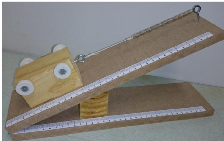
Figura 12 - Imagem da prova experimental da OBFEP 2016
