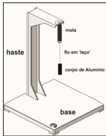
Figura 6 - Imagem da prova experimental da OBFEP 2014
